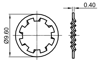
弹垫
