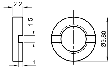
螺母
