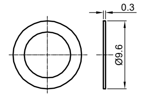
平垫
